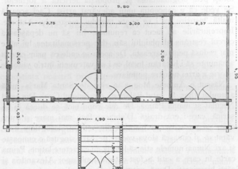
Planul casei lui Mogoș.
