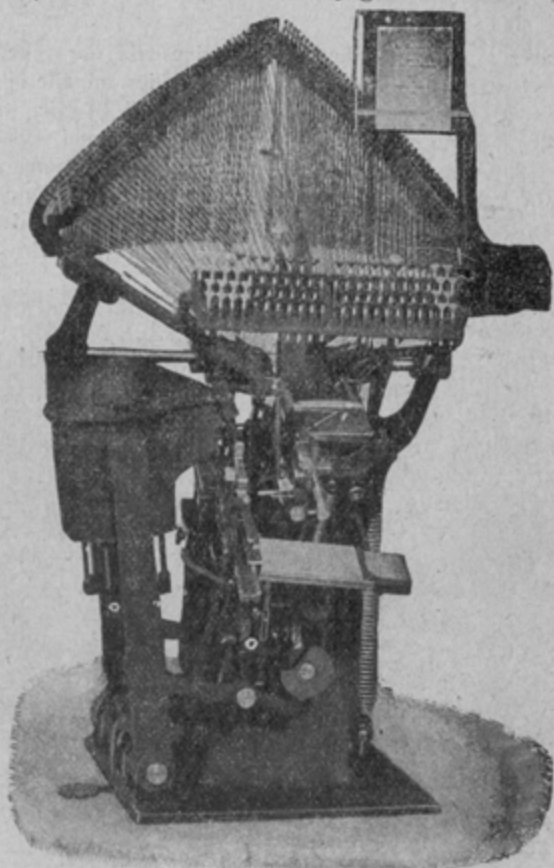
Mașină de cules sistem „Tipograph“.
