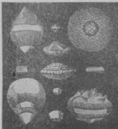
Diferite boabe de grindină.
