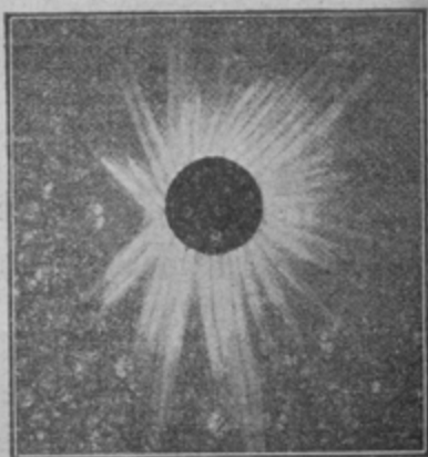
O eclipsă de soare.
