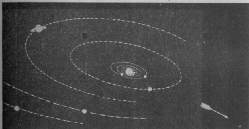
Sistemul solar. — Ansamblul sistemului solar și mișcarea generală în direcția stelei Vega.
