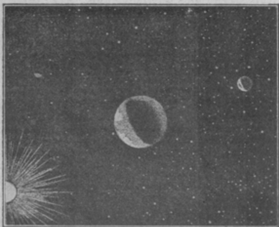
Soarele, pământul, luna. — (Pământul luminat de soare).
