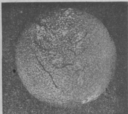
Cromosfera Soarelui. — (Fotografie făcută la observatorul din Meudon).
