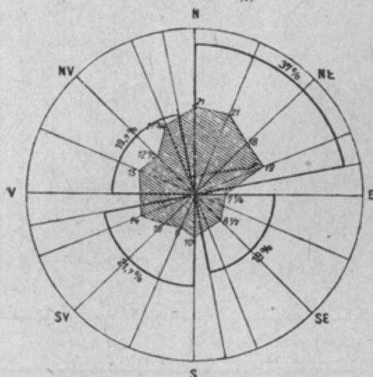
Diagrama direcţiei, duratei şi intensităţii vânturilor la gurile Dunării (Liniste 2,58 ‰)
