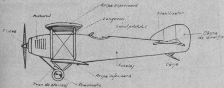
Părțile principale ale avionului.
