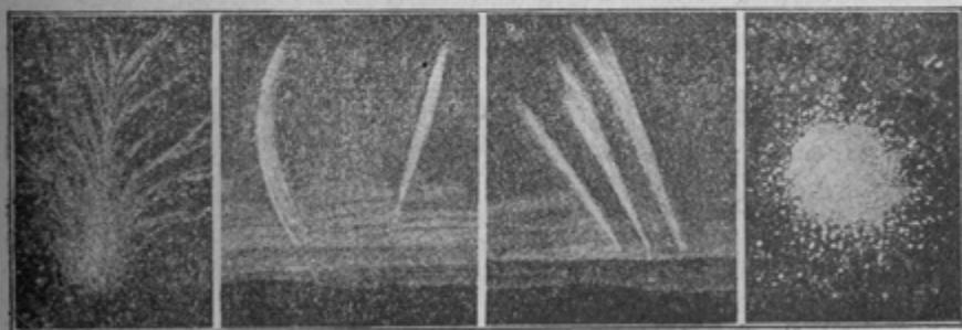
Nebuloasa în formă de „panaș“
