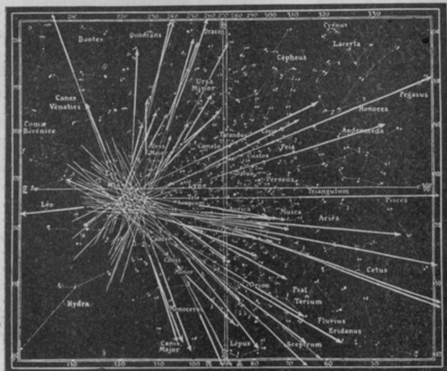
Radiantele stelelor filante. — Punctele de unde par că țâșnesc stelele filante. Convergența traiectoriilor lor e un efect de perspectivă.
