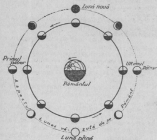
Fazele lunii. — Explicația fazelor lunii.
