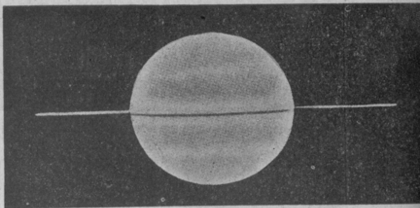
Planeta Saturn cu inelul văzut într'o linie dreaptă.
